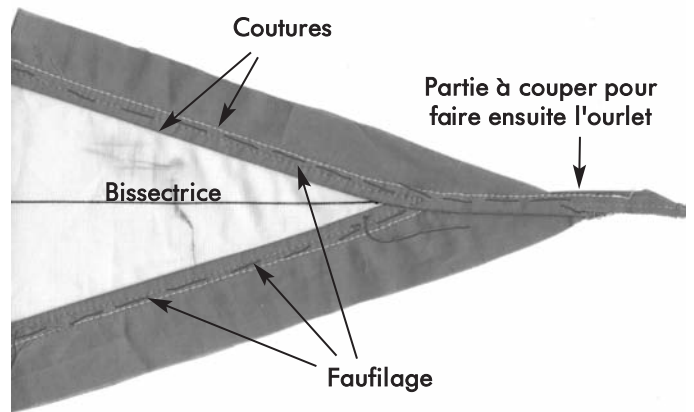
Figure 3 : couture pointe sur l'endroit
